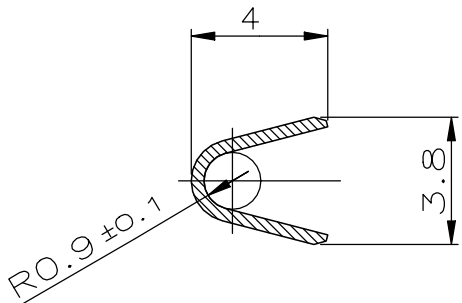
Schnitt B-B SECTION B-B
