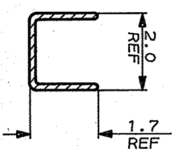
SEZ. (SECT.) E-E
